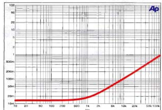
Das Van den Hul mit extrem niedrigem Widerstand (4,65 mΩ/m), aber hoher, von der Verdrehung abhängiger Induktivität (>600 nH/m).
