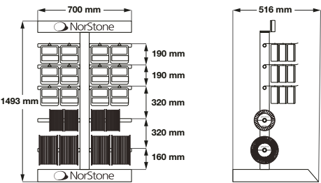
COMBINAISON 2 Packs et rouleaux de câbles Cables packs and rolls assembly
