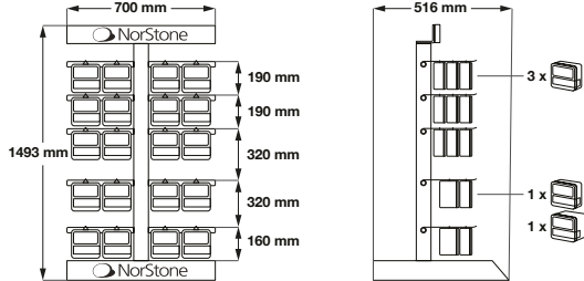
COMBINAISON 1 Packs câbles uniquement Cables packs only
